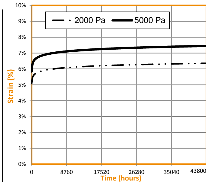
Creep test - EN 1606 (2)
